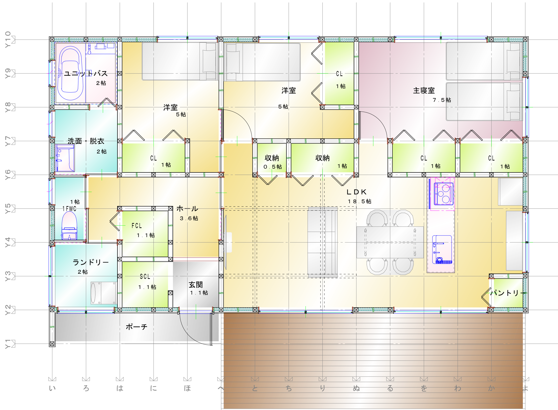
平面詳細図 1階
