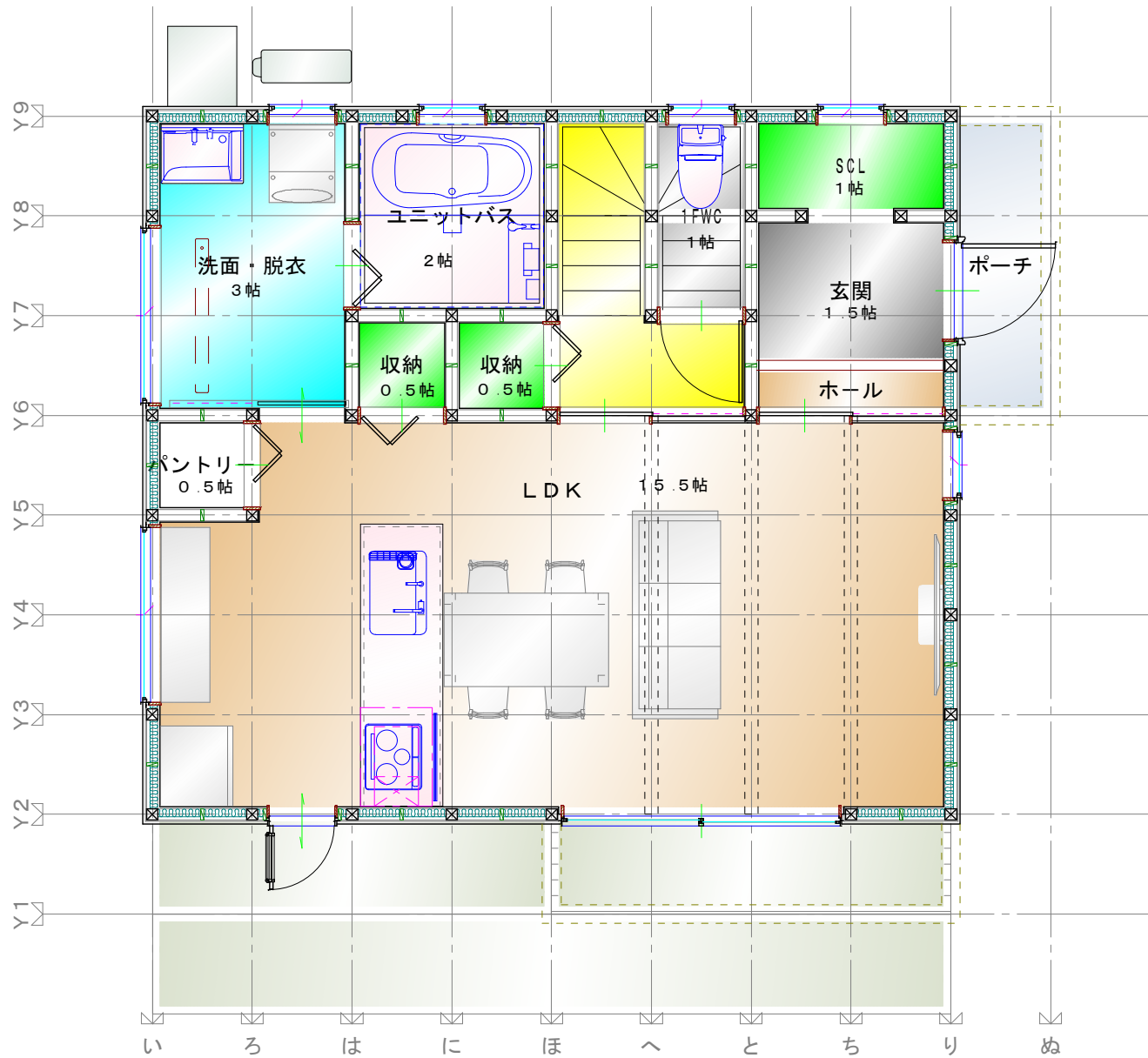
平面詳細図 1階
