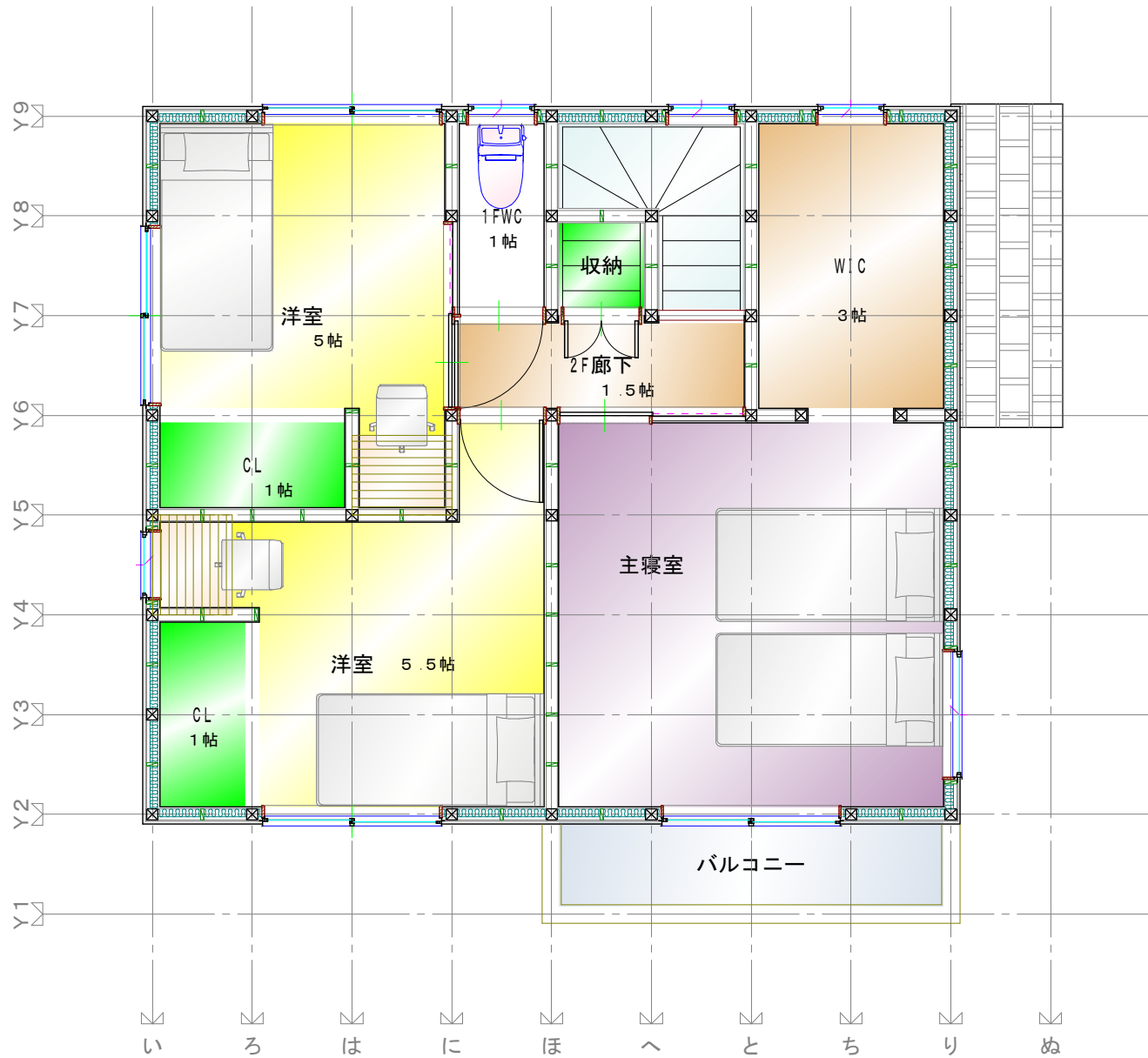
平面詳細図 2階
